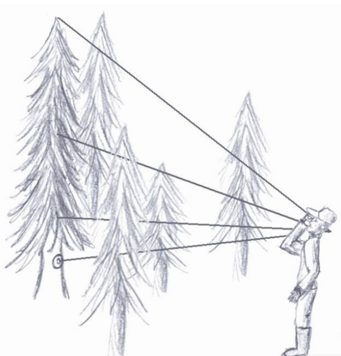
Hình 04. Đo chiều cao vút ngọn của cây bằng thước đo cao Vertex
